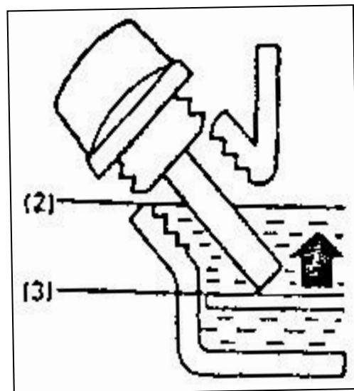
Рис. 14. Нормальный уровень масла
